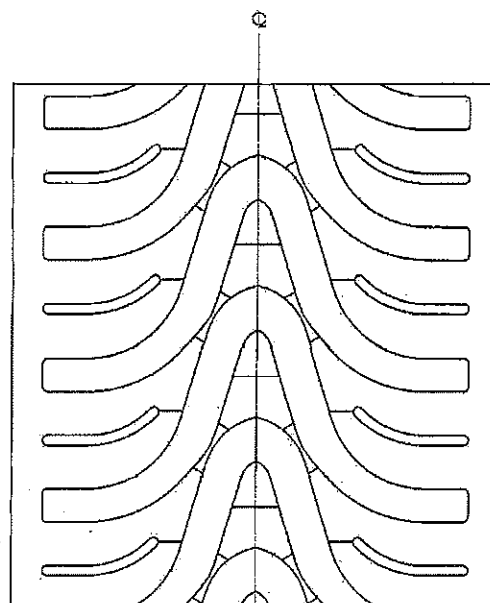
DESSIN DE LA BANDE DE ROULEMENT TREAD DESIGN DRAWING
